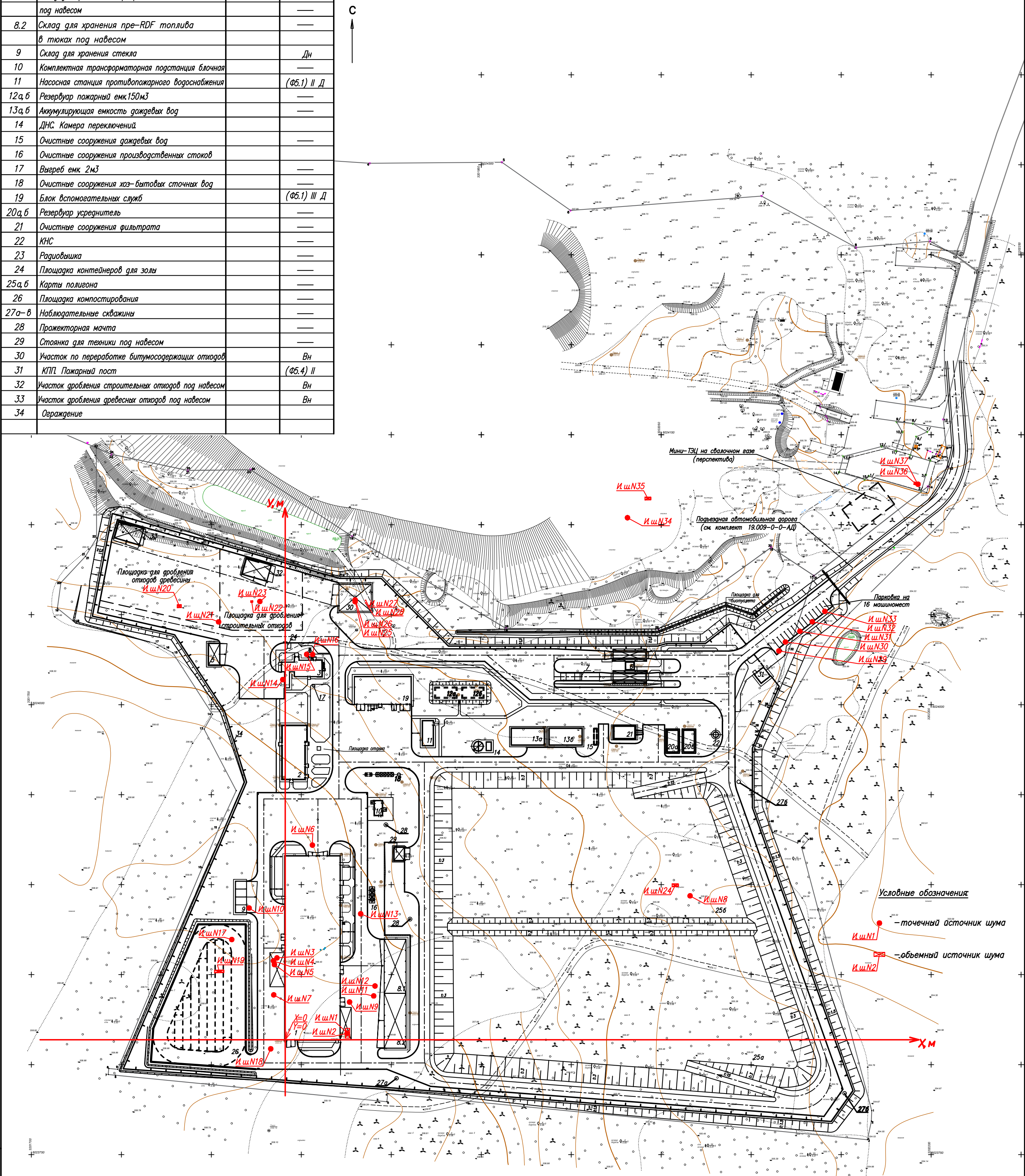
Генплан с источниками шума (1:1000)
