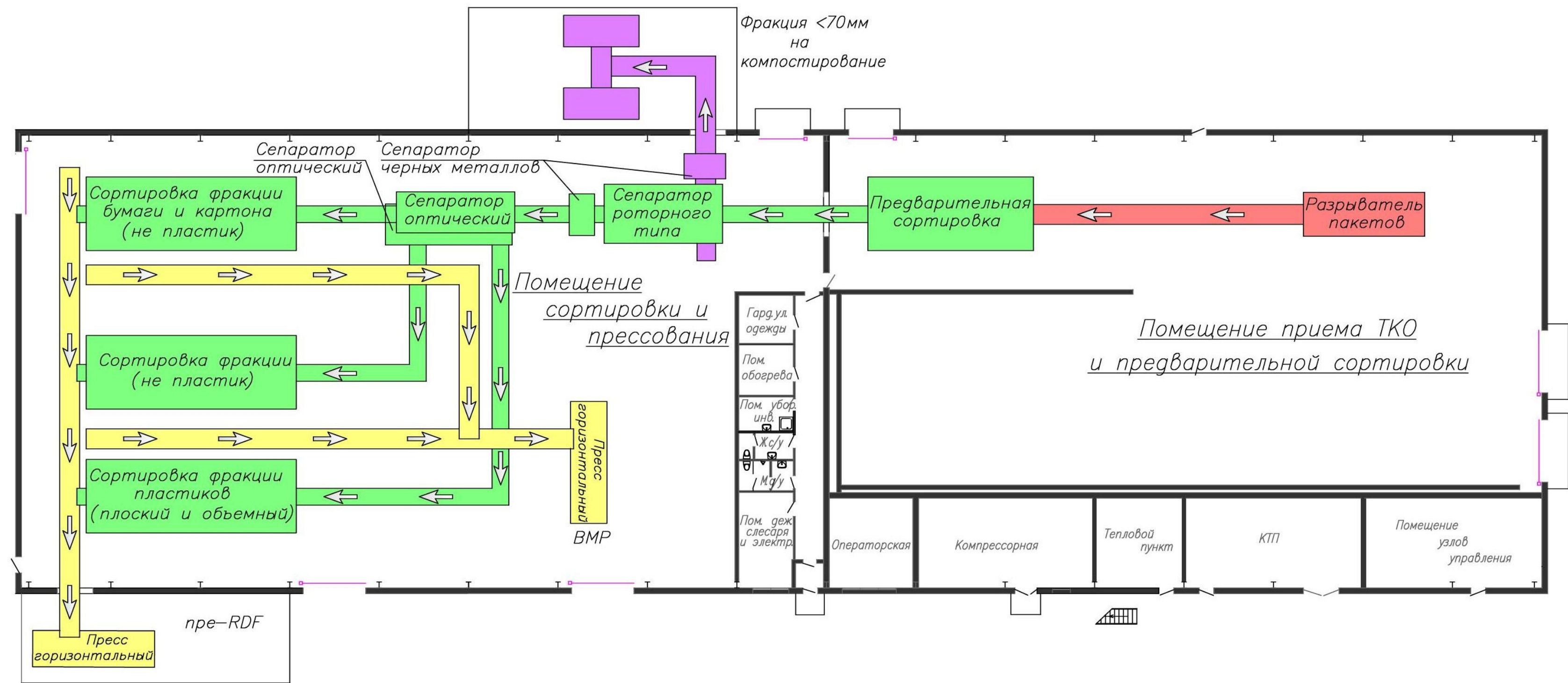
Рис.2.2. Технологическая схема
