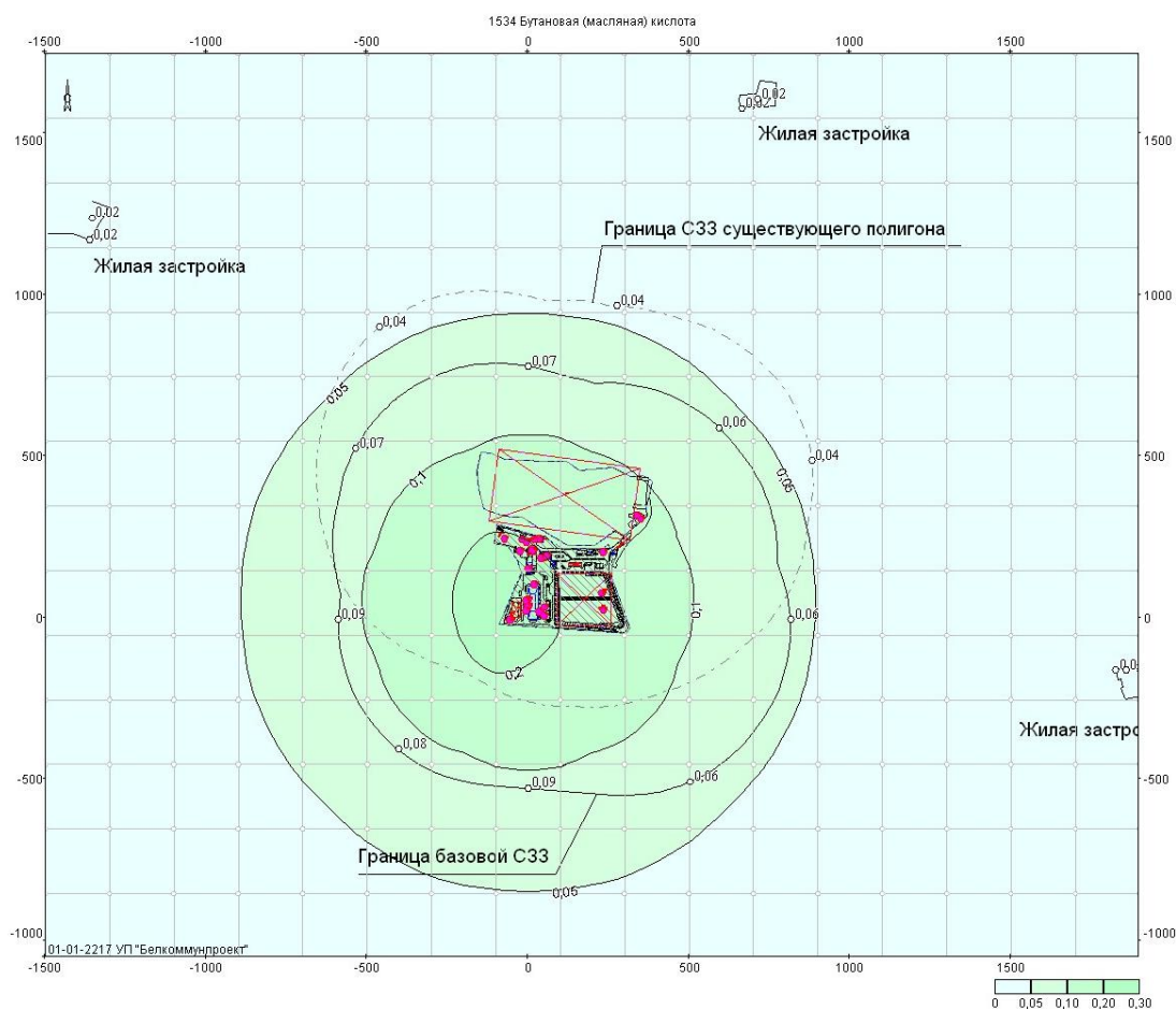
Рис. 5.2. Карта изолиний расчетных концентраций бутановой кислоты
