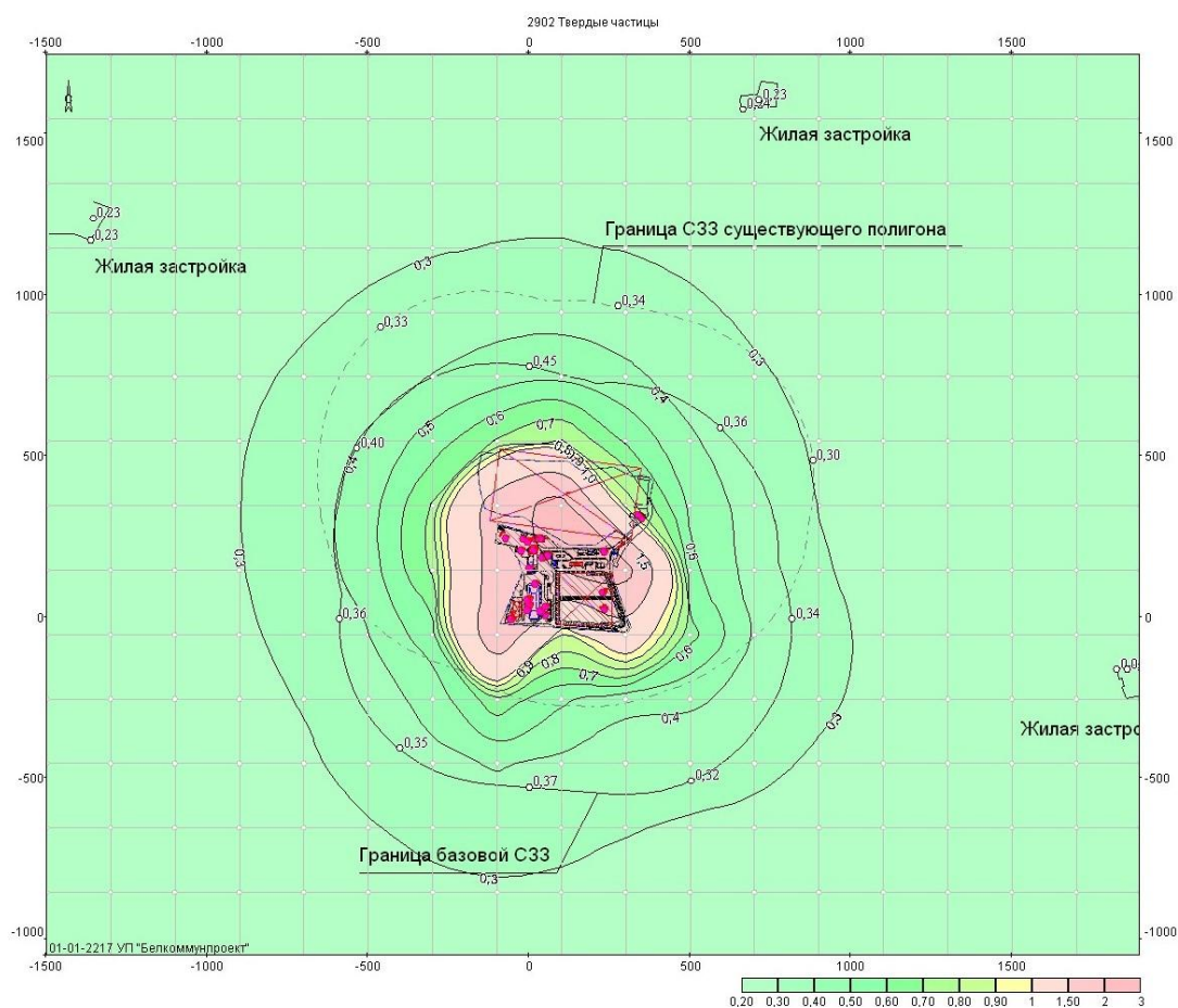
Рис. 5.3. Карта изолиний расчетных концентраций твердых частиц
