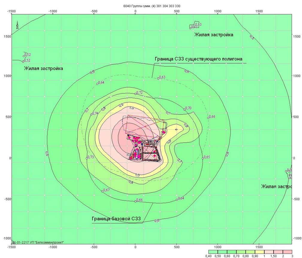
Рис. 5.5. Карта изолиний расчетных концентраций группы суммации 6040
