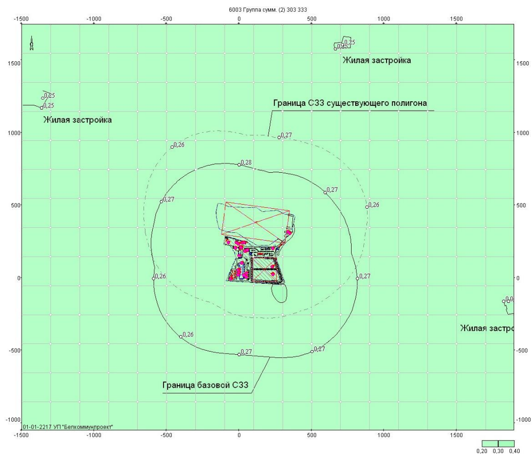
Рис. 5.4. Карта изолиний расчетных концентраций группы суммации 6003
