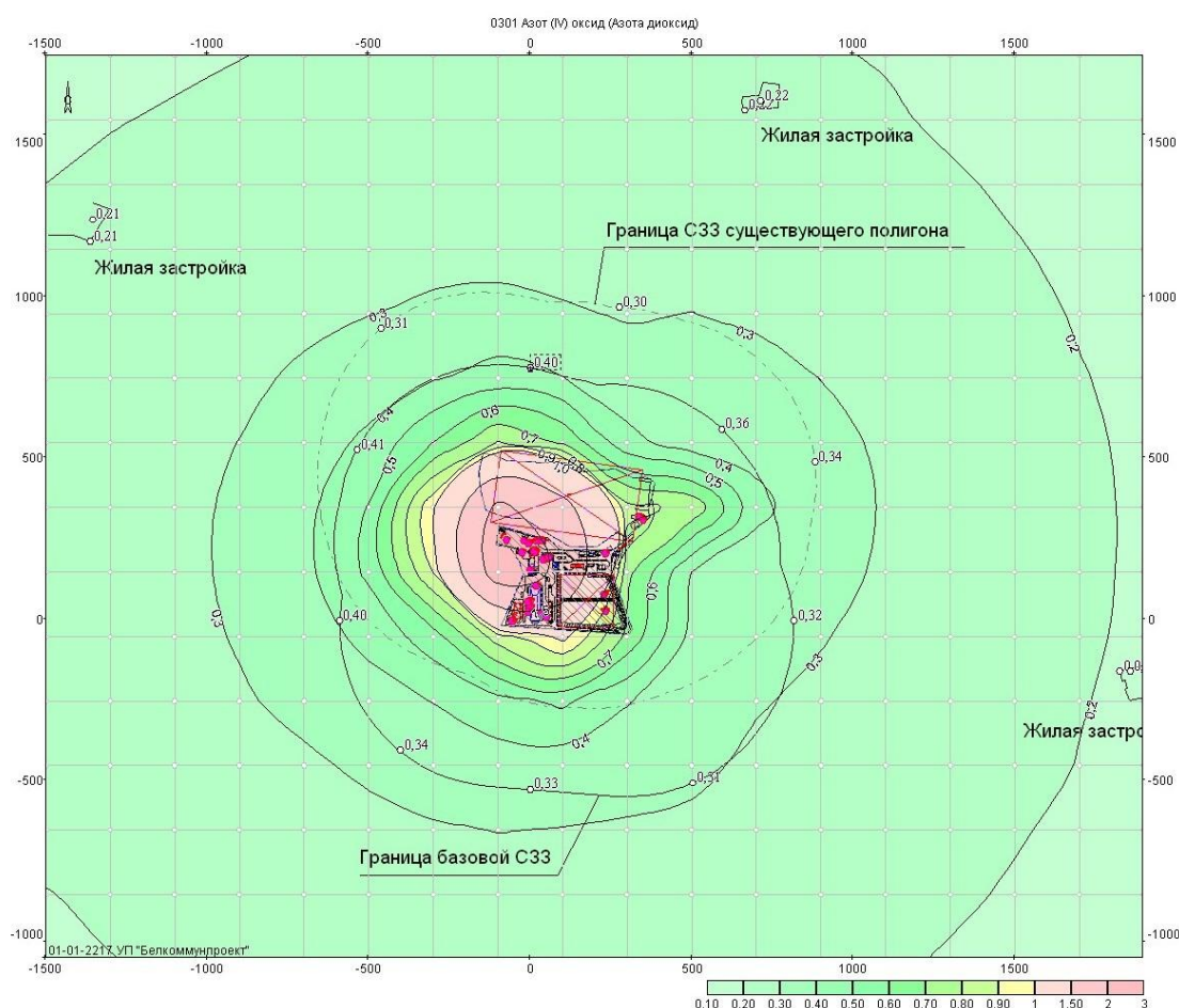
Рис. 5.1. Карта изолиний расчетных концентраций азота диоксида
